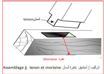
Assemblage à tenon et mortaise تشبيك بنقرة ولسان
