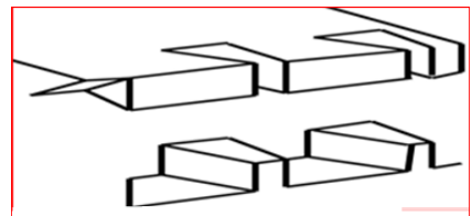
Assemblage embrèvement carré
