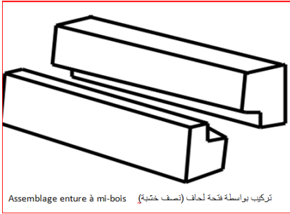
Assemblage trave carré
