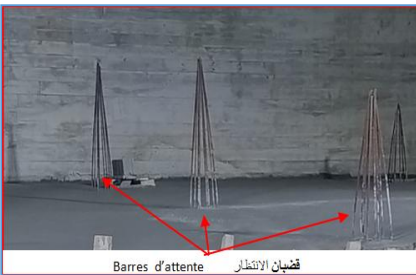
Barres d'attente قضبان الانتظار
