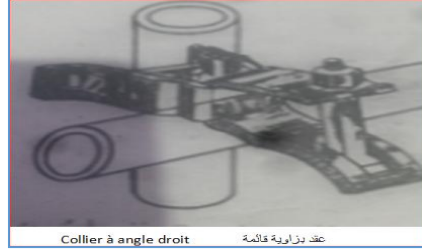
Collier à angle droit عقد بزواية قائمة
