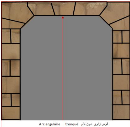
قوس زاوي دون تاج
