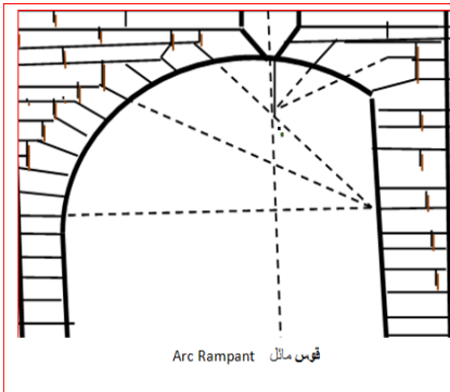
Arc Rampant قوس مائل
