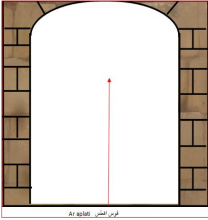
Arc en doucine قوس ظهر الحمار
