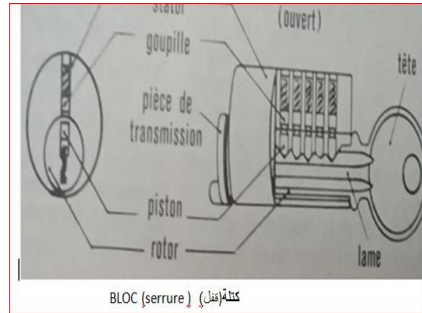
BLOC (serrure) كتلة (قفل)
