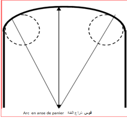
Arc-boutant
